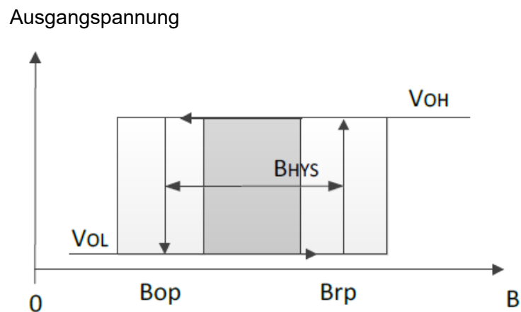
Ausgangsverhalten von CYD511
